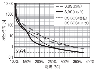
● 形 R88M-1M20030T
