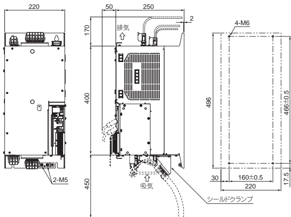
外形寸法
