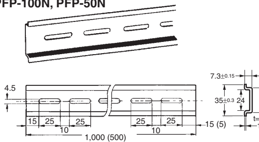
PFP-100N, PFP-50N
