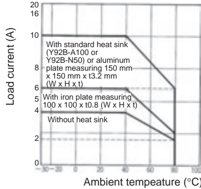
G3NA-240B-UTU
