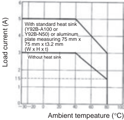
G3NA-225B-UTU G3NA-425B-UTU-2
